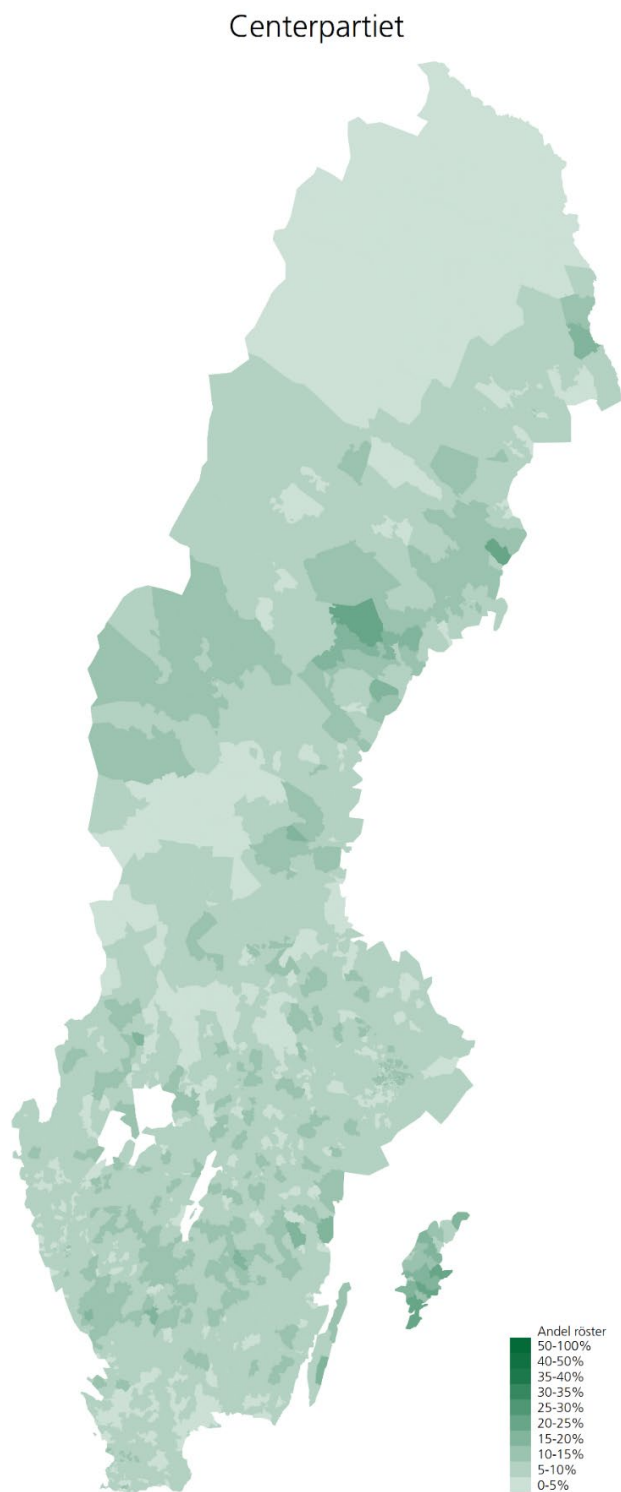
Figur A.9 Centerpartiets röststöd i 2022 års riksdagsval (procent).
