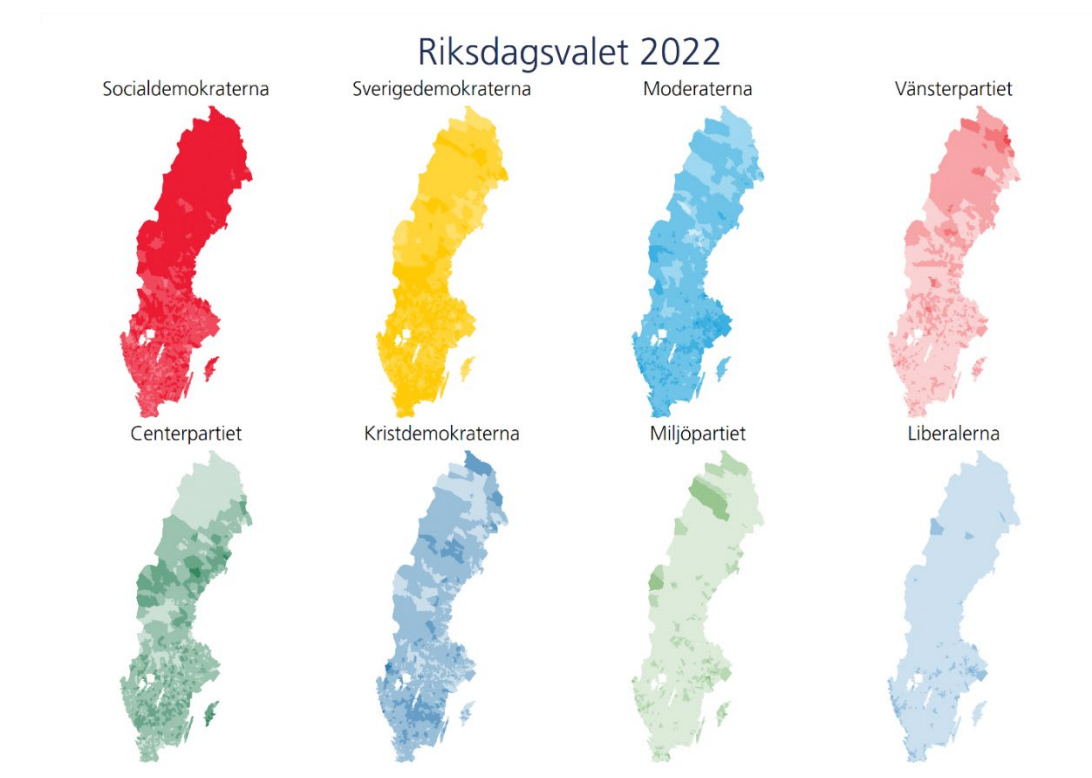
Figur 6 Partiernas procentuella röststöd i landets 6 264 valdistrikt i 2022 års riksdagsval.
