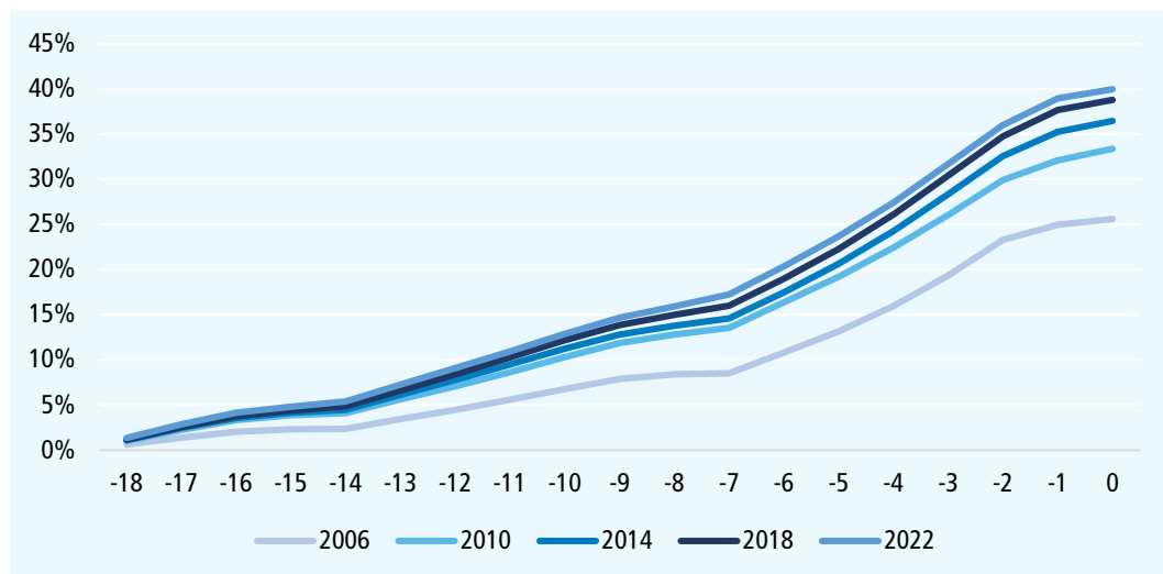
Figur 1 Inströmning av förtida röster i svenska val 2006–2022 under de sista 18 dagarna före valet (ackumulerad andel) Absentee voting in Swedish elections 2006–2022 the last 18 days before Election Day (accumulated proportions).
