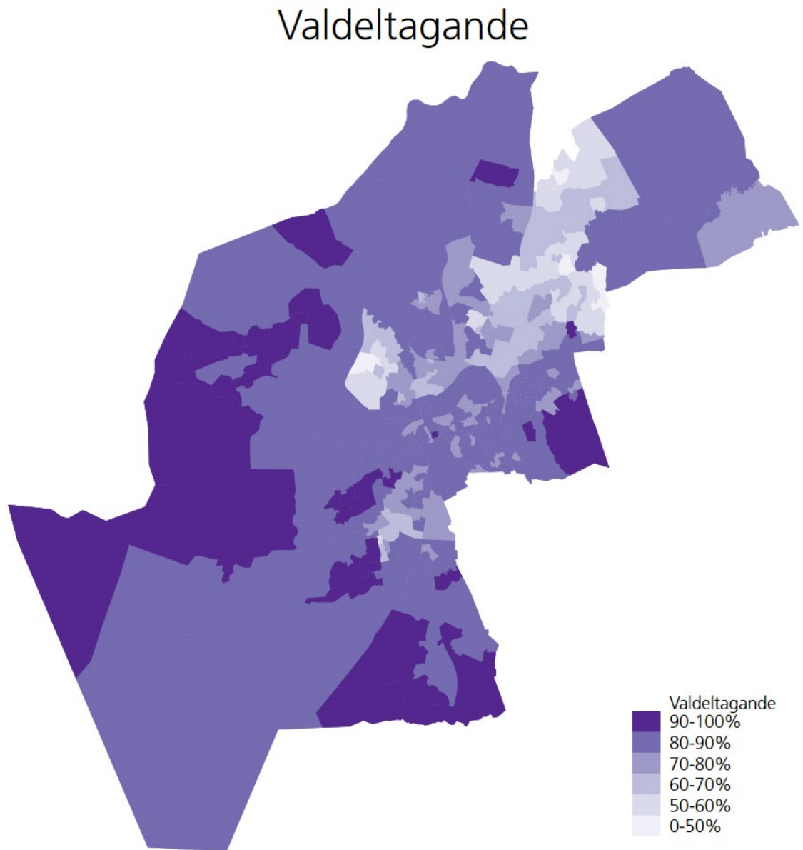
Figur A.3 Valdeltagandet i Göteborgs valdistrikt i 2022 års riksdagsval (procent).
