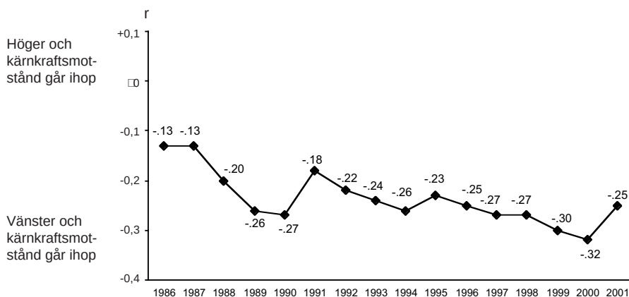
Figur 3 Sambandet mellan väljarnas kärnkraftsåsikter och självuppskattad vänster-högerposition (r)
